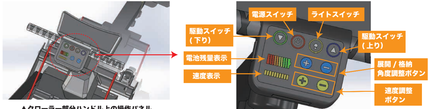
▲クローラー部分ハンドル上の操作パネル
